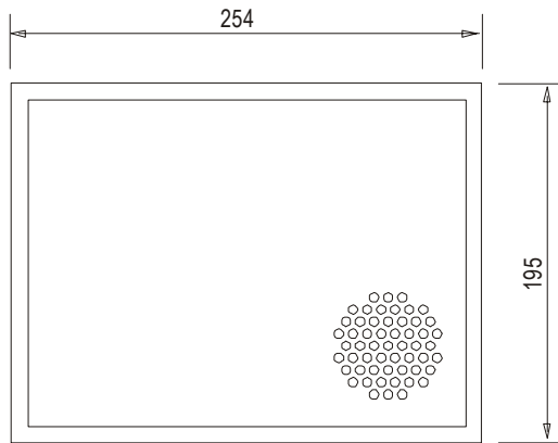
Frontansicht
