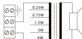
Leistungsanschlussbelegung (2x)
