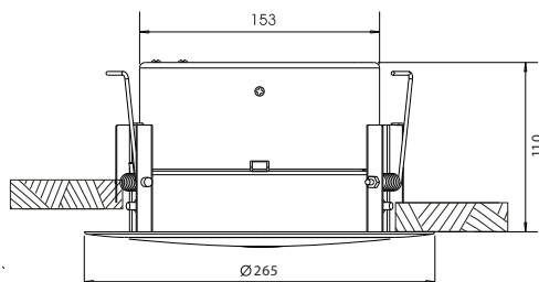
RGS 8/FTS a/b Seitenansicht
