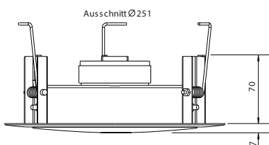
RGS 8/T a/b Seitenansicht
