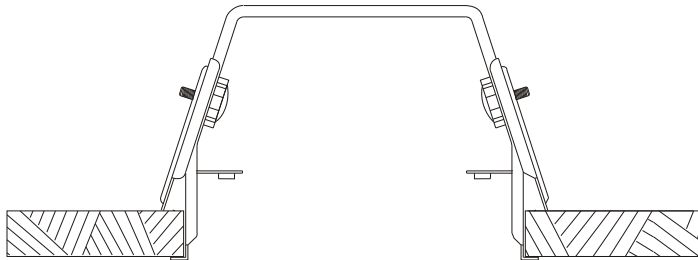
Ausschnitt für RCS 8/T = 236 mm
